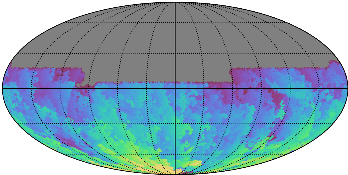
baseline_v3.3_10yrs All sky u band: Max HA
