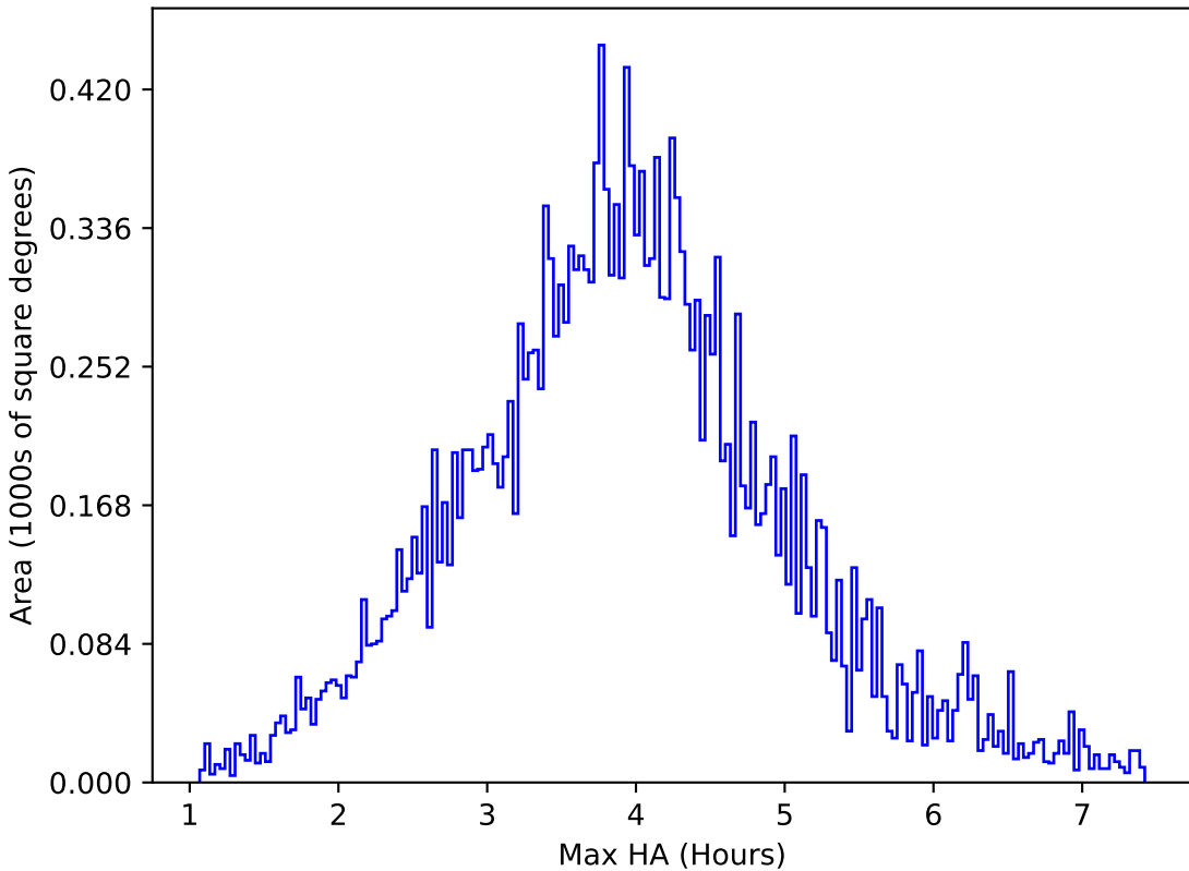
baseline_v3.3_10yrs All sky u band: Max HA
