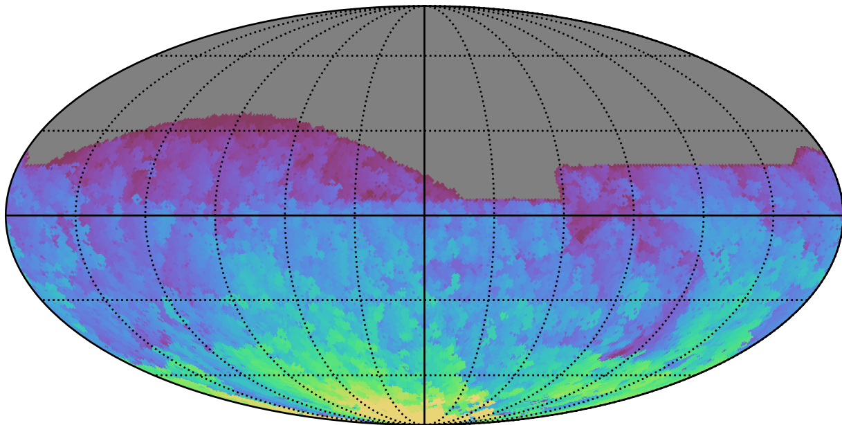
baseline_v3.3_10yrs All sky r band: Max HA
