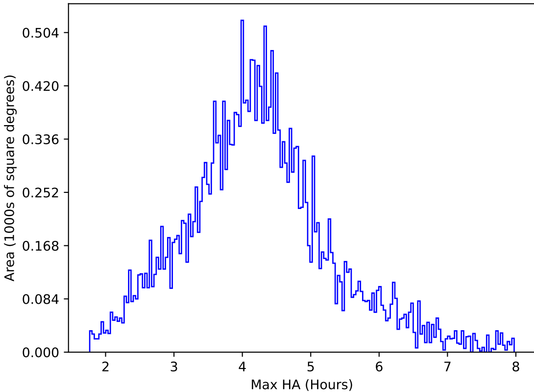
baseline_v3.3_10yrs All sky r band: Max HA
