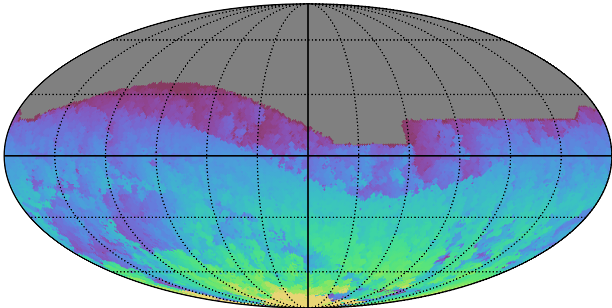
baseline_v3.3_10yrs All sky i band: Max HA
