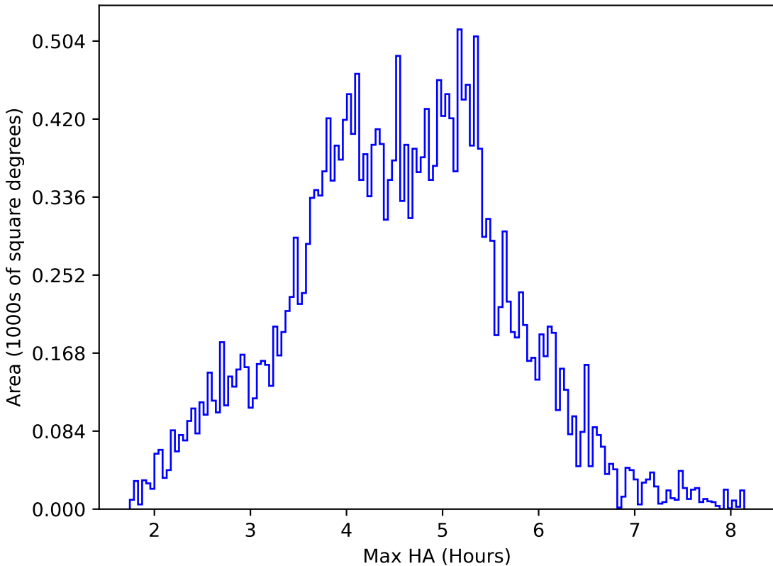
baseline_v3.3_10yrs All sky i band: Max HA
