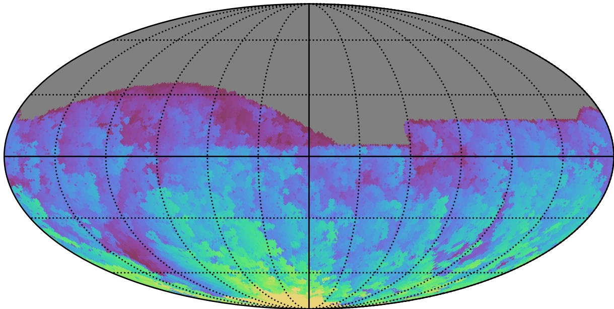
baseline_v3.3_10yrs All sky g band: Max HA
