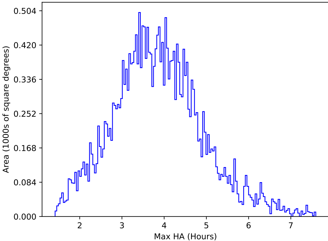
baseline_v3.3_10yrs All sky g band: Max HA
