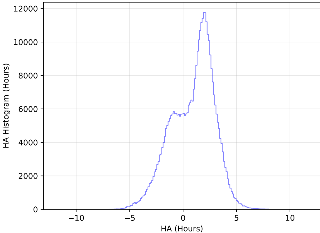
baseline_v3.3_10yrs WFD y band: HA Histogram
