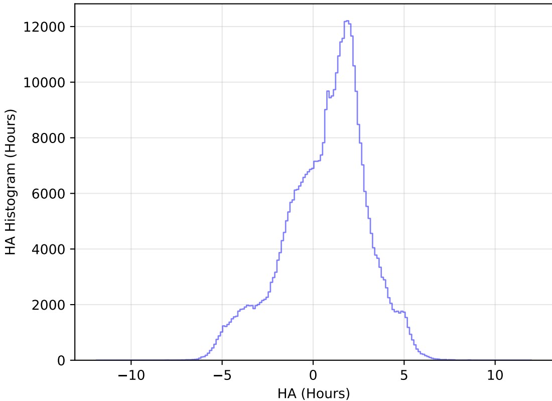
baseline_v3.3_10yrs All sky z band: HA Histogram
