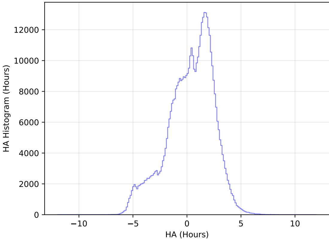
baseline_v3.3_10yrs All sky r band: HA Histogram
