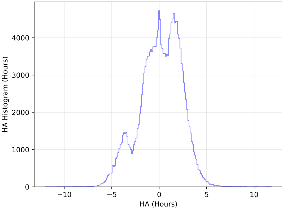
baseline_v3.3_10yrs All sky g band: HA Histogram
