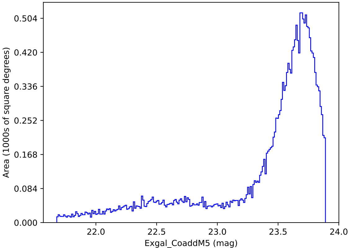
baseline_v3.3_10yrs Yr 1 y band: Exgal_CoaddM5
