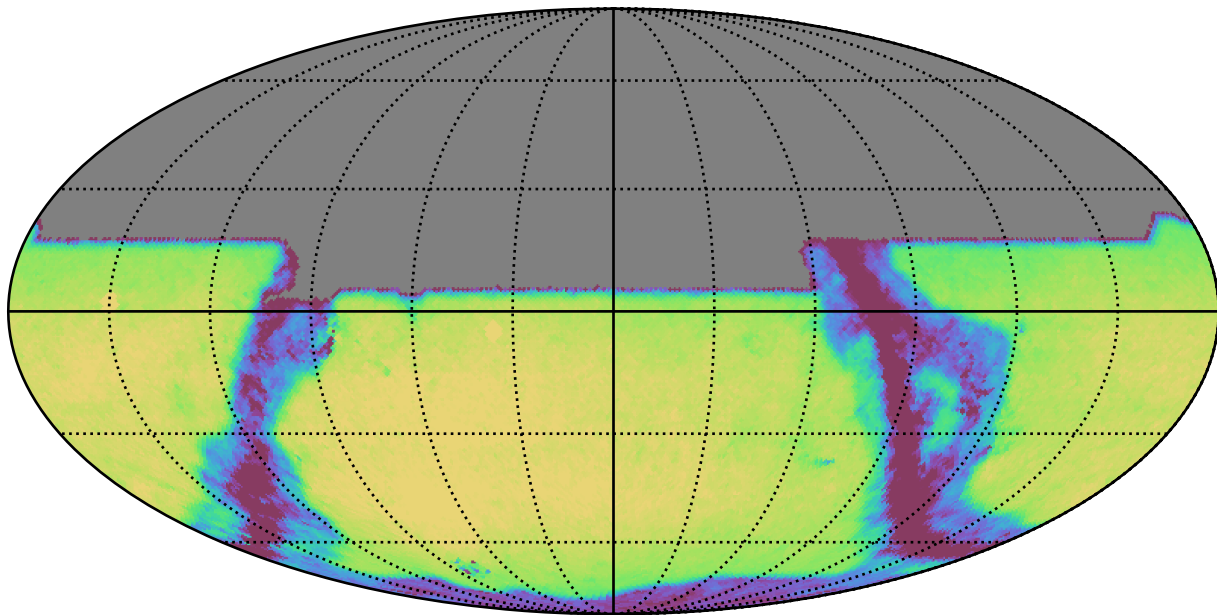
baseline_v3.3_10yrs All sky y band: Exgal_CoaddM5
