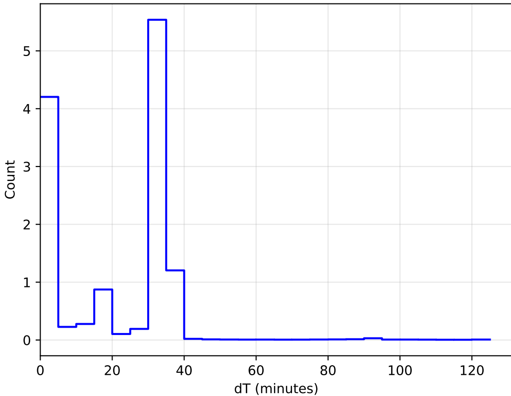
1e6 baseline_v3.3_10yrs All sky: DeltaT Histogram
