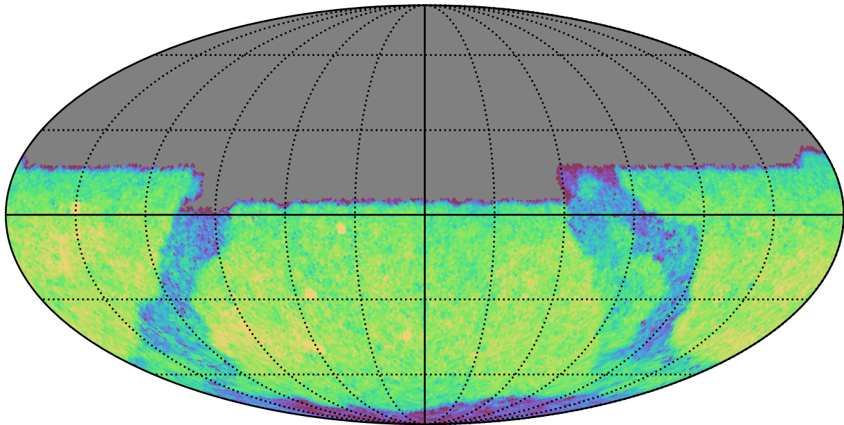
baseline_v3.3_10yrs Yr 1 y band: CoaddM5
