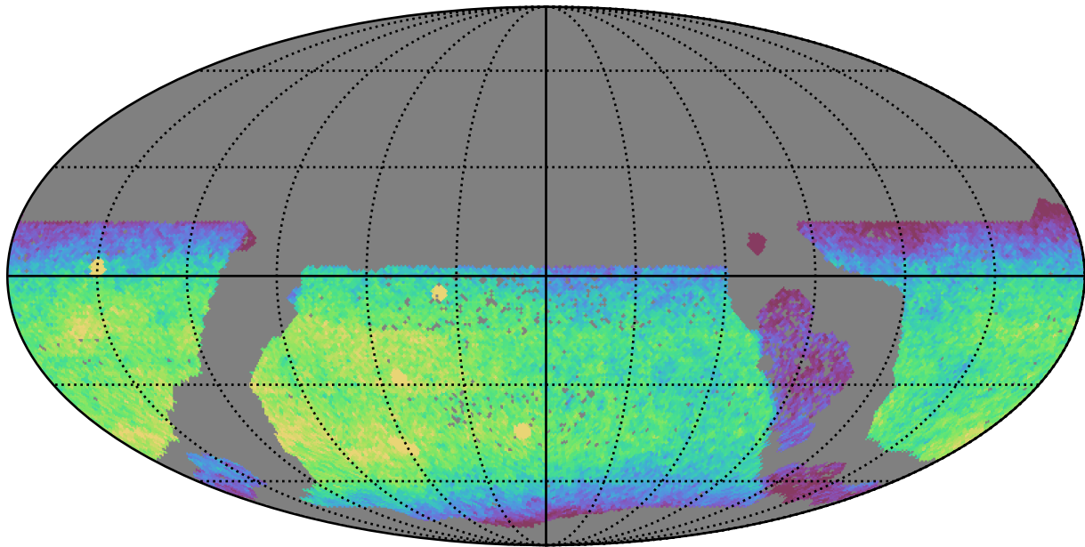
baseline_v3.3_10yrs WFD y band: CoaddM5
