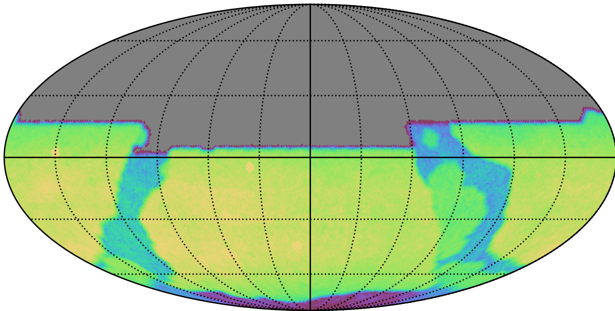
baseline_v3.3_10yrs All sky y band: CoaddM5
