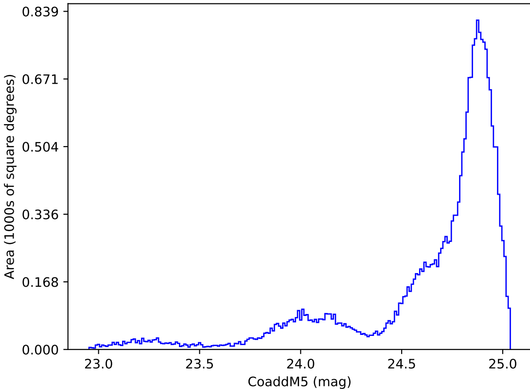
baseline_v3.3_10yrs All sky y band: CoaddM5
