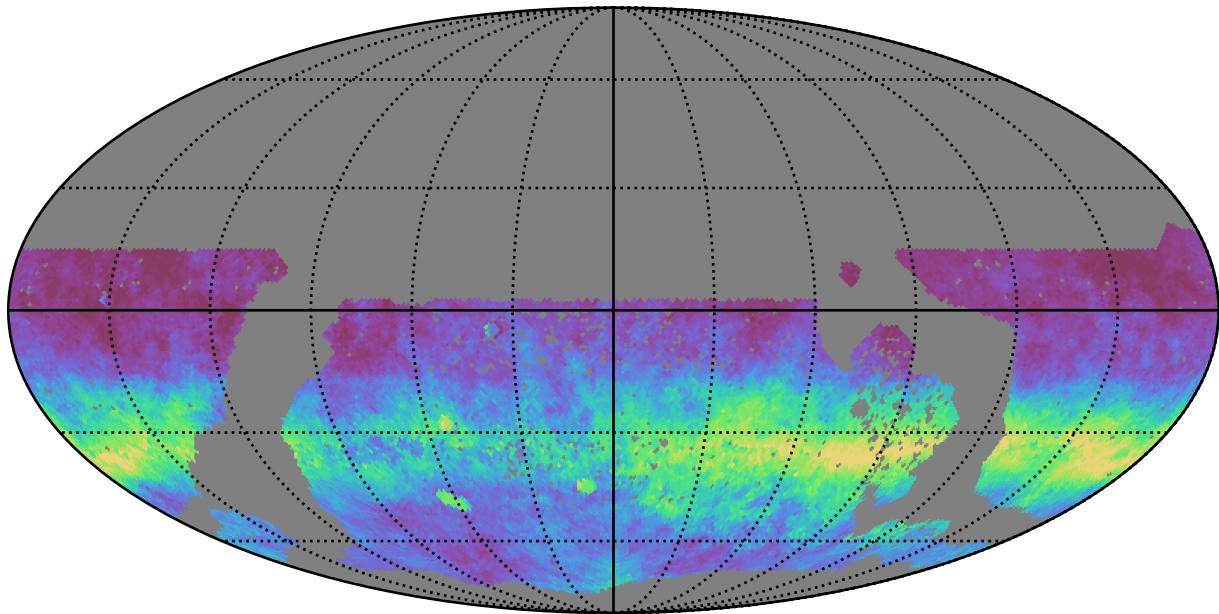
baseline_v3.3_10yrs WFD z band: AngleRms rotSkyPos
