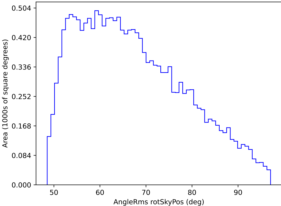
baseline_v3.3_10yrs WFD z band: AngleRms rotSkyPos
