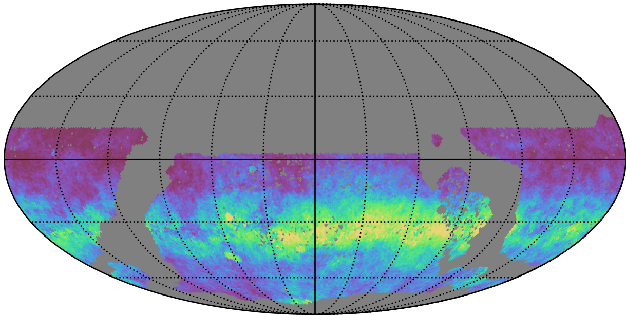
baseline_v3.3_10yrs WFD y band: AngleRms rotSkyPos
