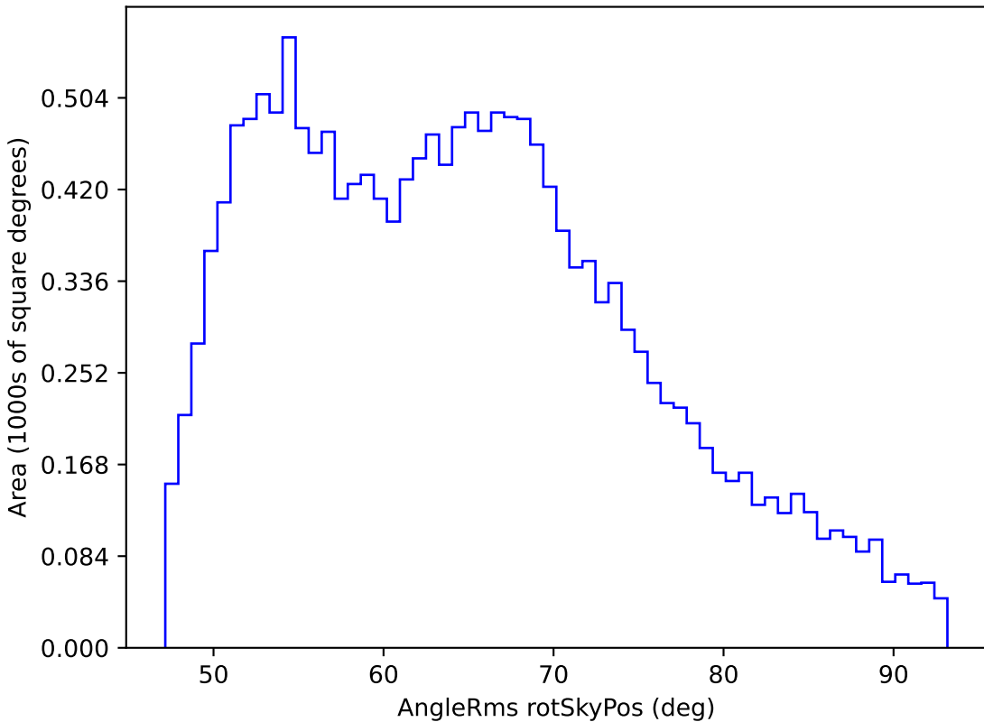
baseline_v3.3_10yrs WFD y band: AngleRms rotSkyPos
