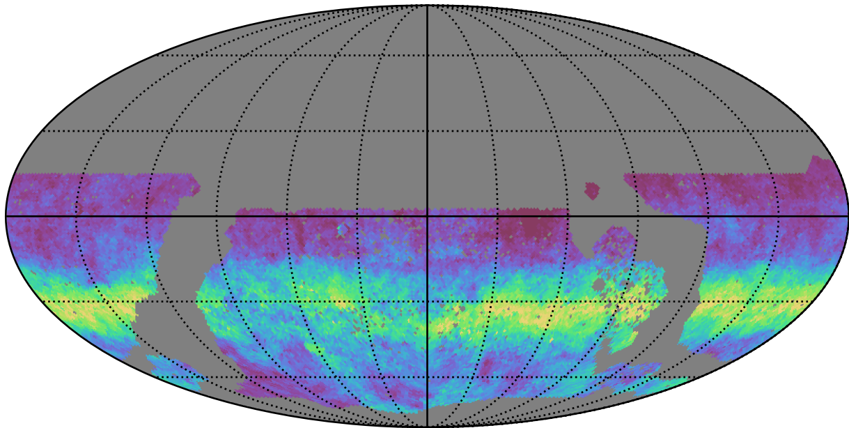
baseline_v3.3_10yrs WFD u band: AngleRms rotSkyPos
