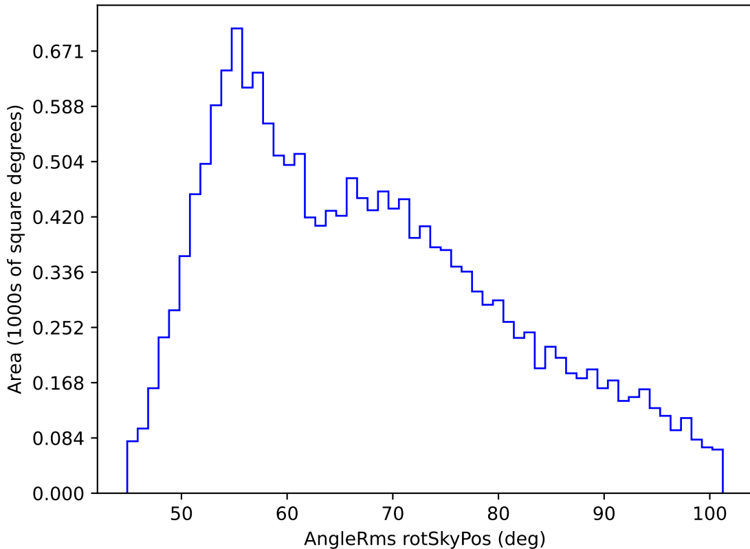
baseline_v3.3_10yrs WFD u band: AngleRms rotSkyPos
