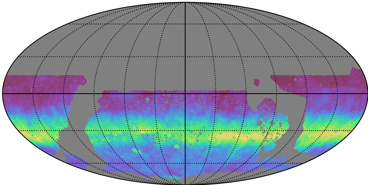
baseline_v3.3_10yrs WFD r band: AngleRms rotSkyPos
