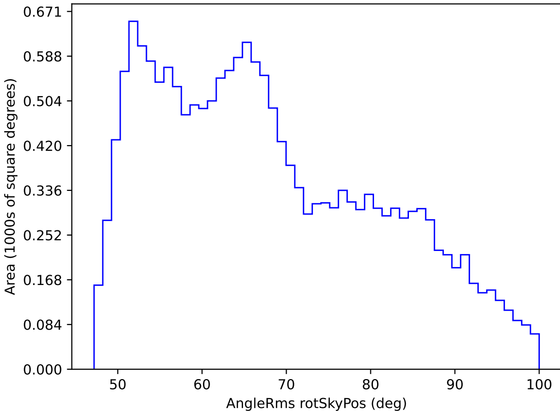
baseline_v3.3_10yrs WFD r band: AngleRms rotSkyPos
