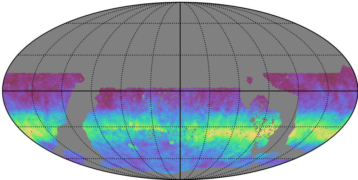
baseline_v3.3_10yrs WFD i band: AngleRms rotSkyPos
