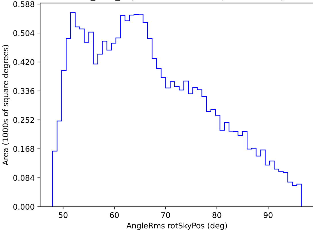
baseline_v3.3_10yrs WFD i band: AngleRms rotSkyPos
