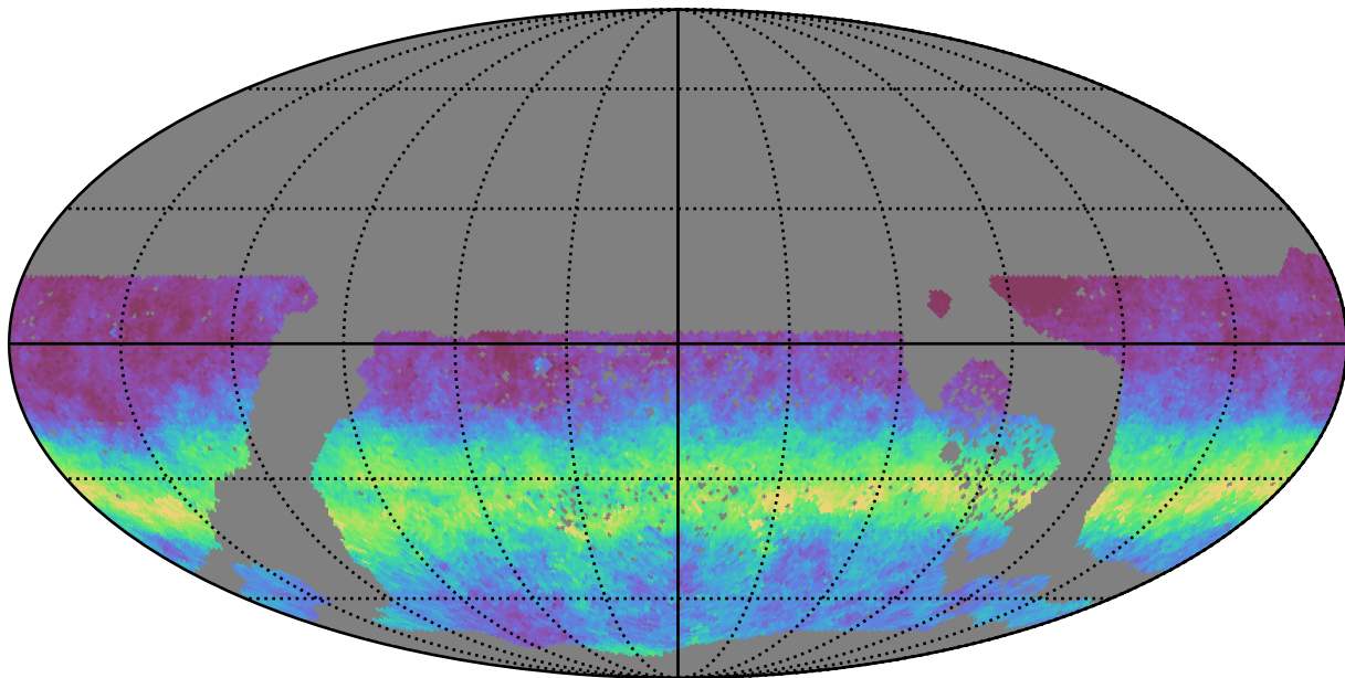
baseline_v3.3_10yrs WFD g band: AngleRms rotSkyPos
