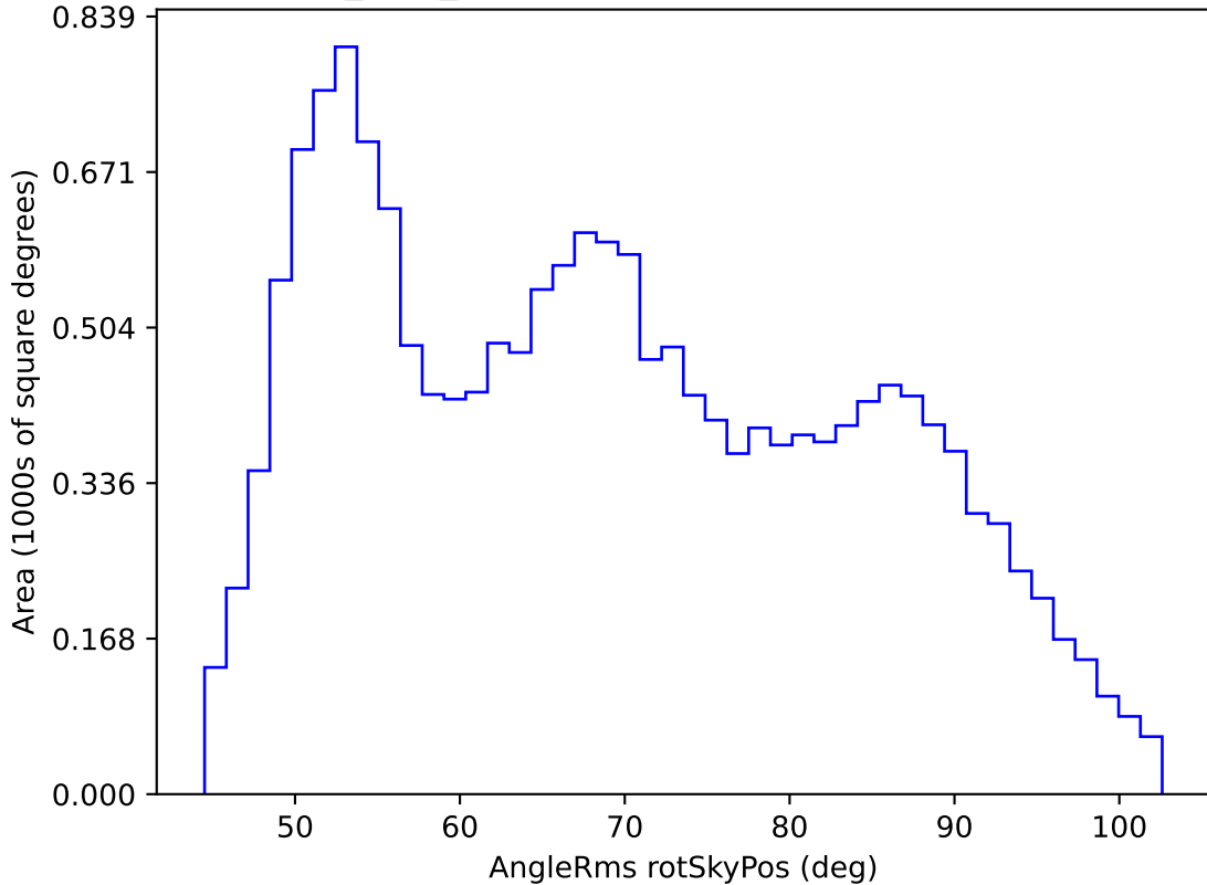
baseline_v3.3_10yrs WFD g band: AngleRms rotSkyPos
