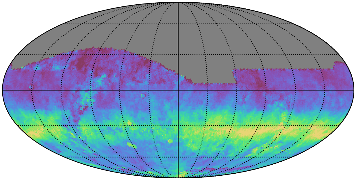
baseline_v3.3_10yrs All sky z band: AngleRms rotSkyPos
