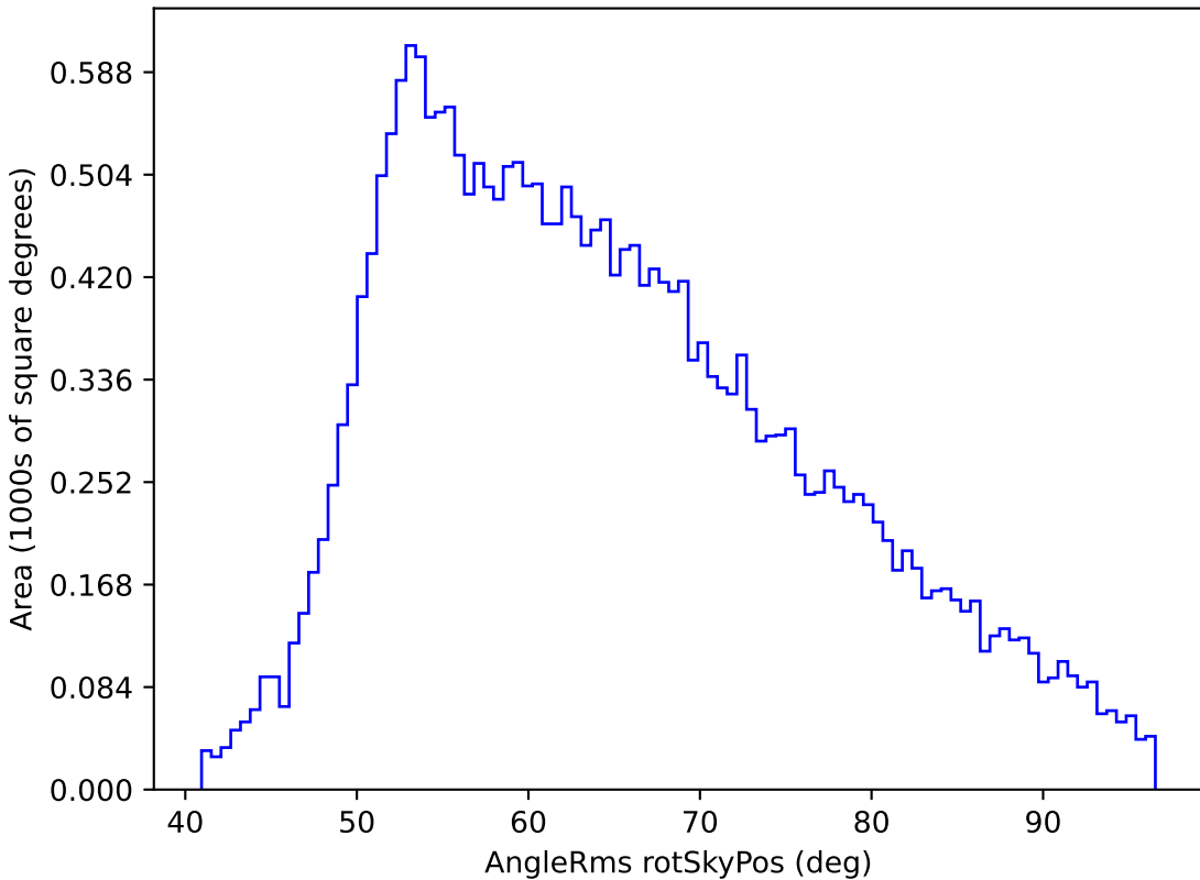
baseline_v3.3_10yrs All sky z band: AngleRms rotSkyPos
