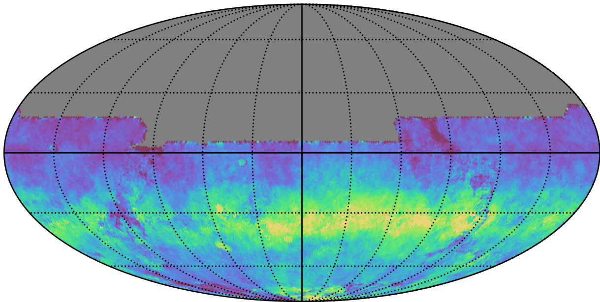
baseline_v3.3_10yrs All sky y band: AngleRms rotSkyPos
