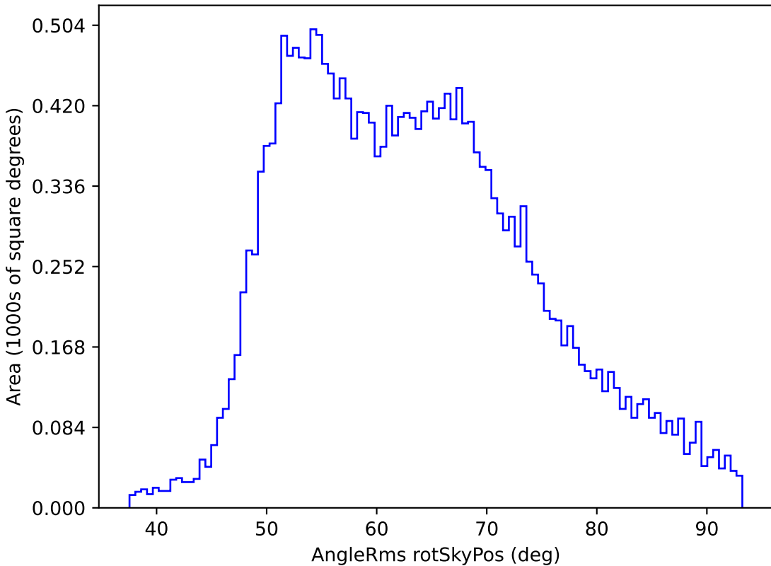
baseline_v3.3_10yrs All sky y band: AngleRms rotSkyPos
