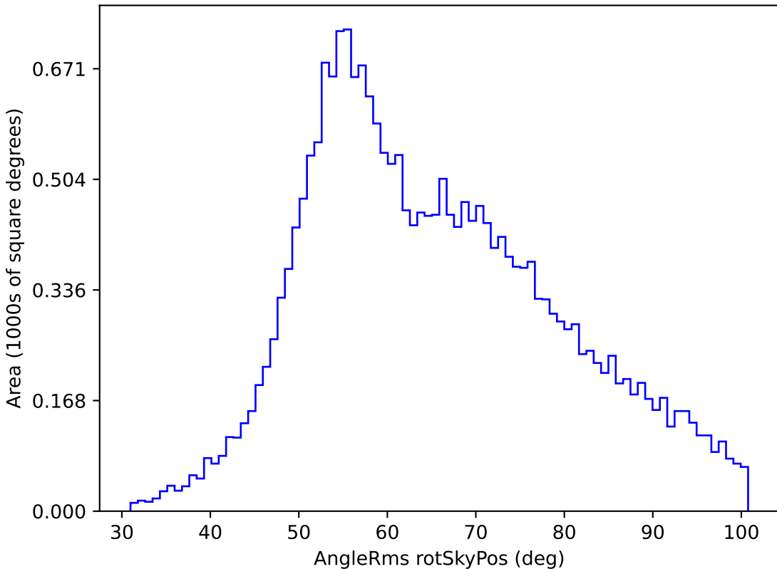
baseline_v3.3_10yrs All sky u band: AngleRms rotSkyPos
