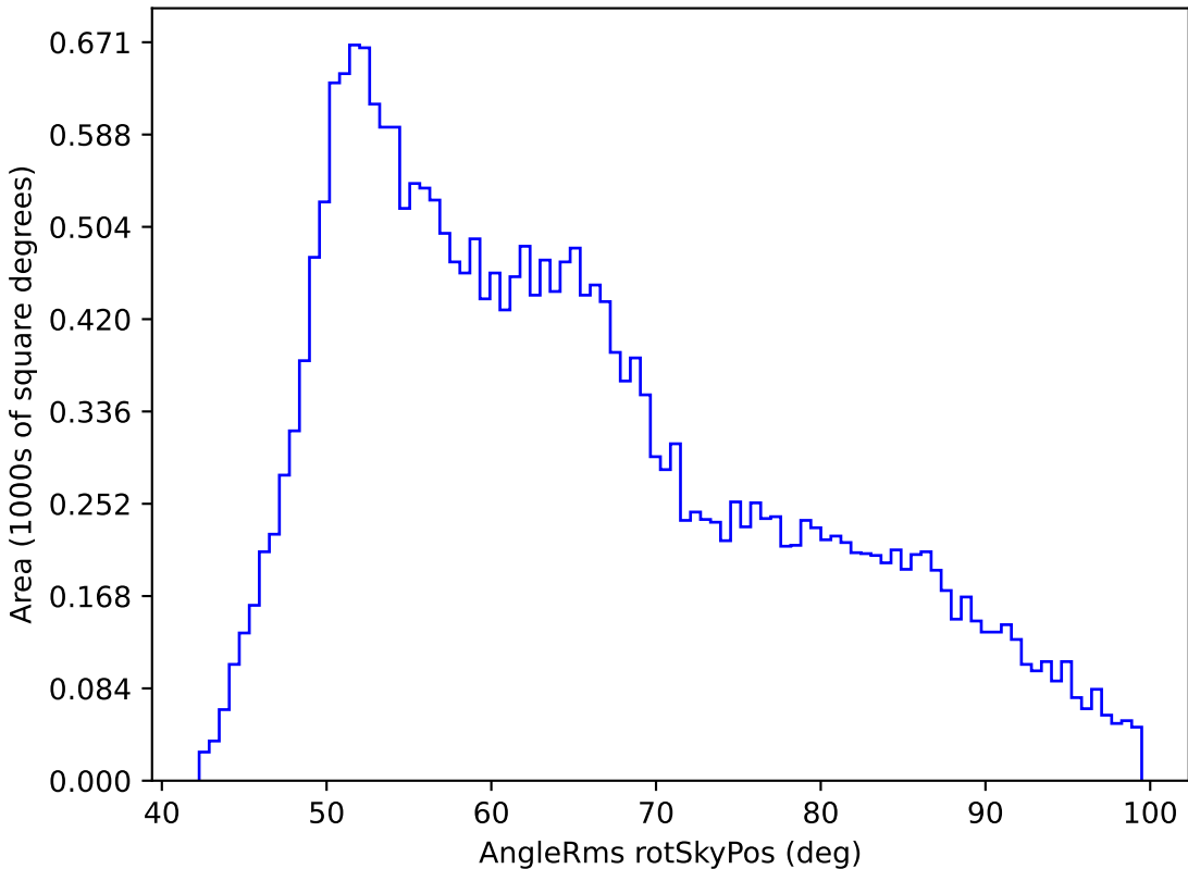
baseline_v3.3_10yrs All sky r band: AngleRms rotSkyPos
