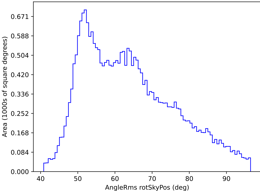
baseline_v3.3_10yrs All sky i band: AngleRms rotSkyPos
