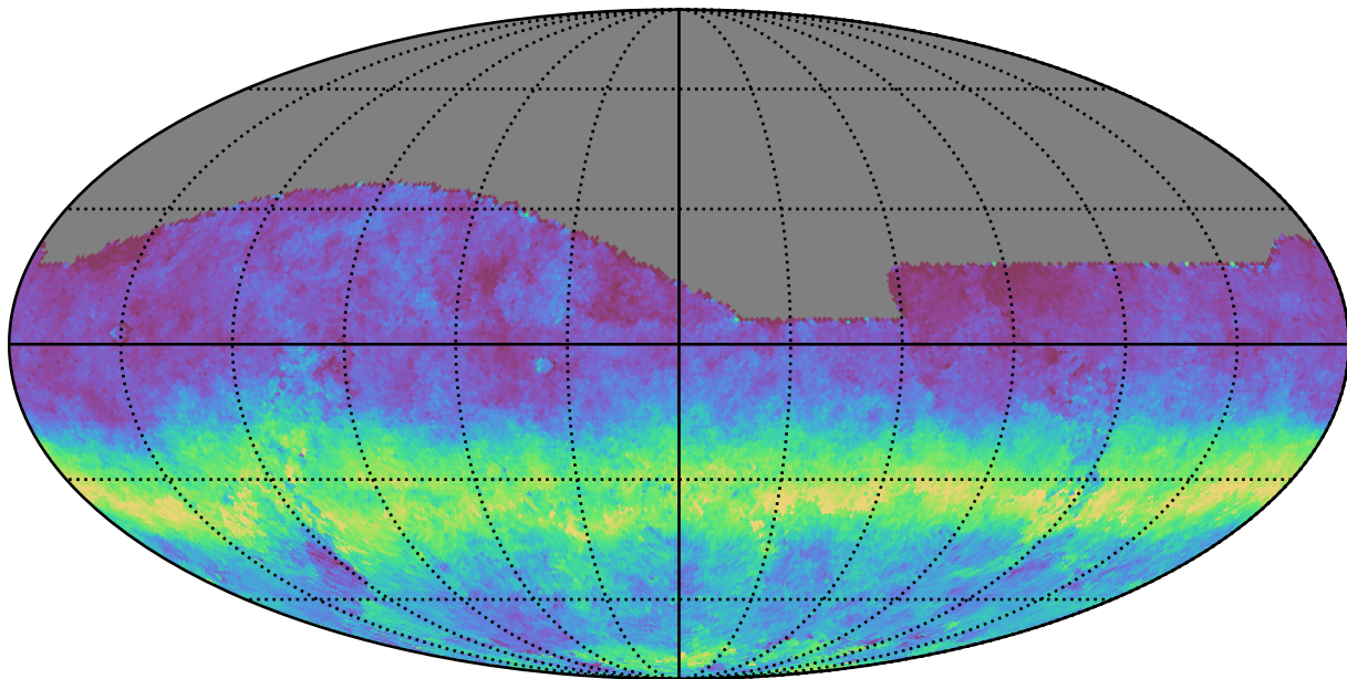
baseline_v3.3_10yrs All sky g band: AngleRms rotSkyPos
