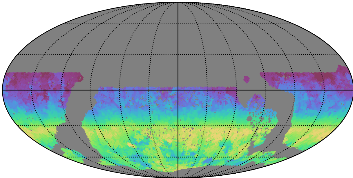
baseline_v3.3_10yrs WFD z band: AngleRange rotSkyPos
