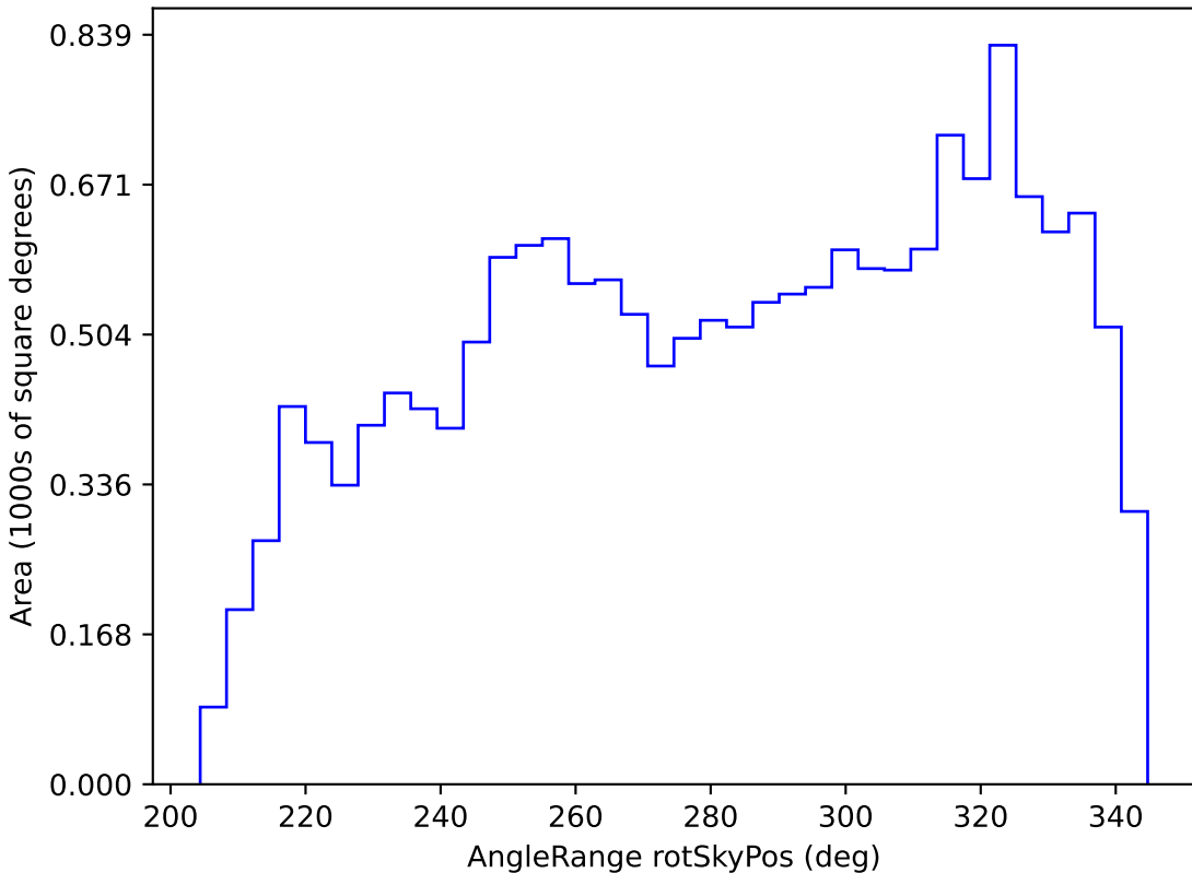
baseline_v3.3_10yrs WFD z band: AngleRange rotSkyPos
