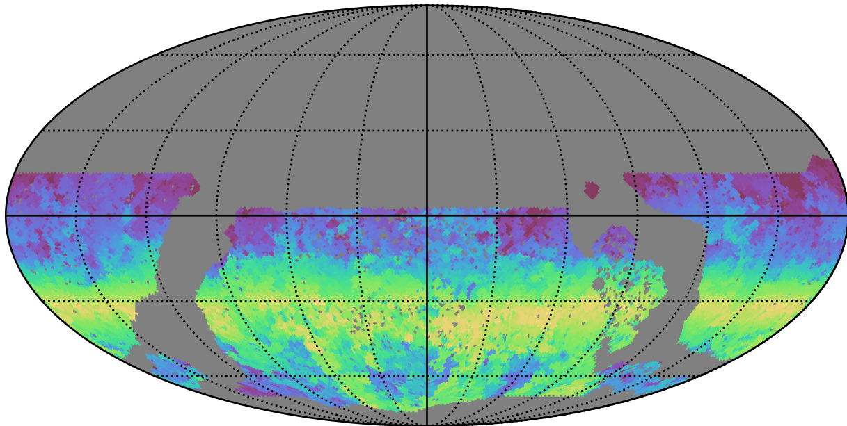
baseline_v3.3_10yrs WFD u band: AngleRange rotSkyPos
