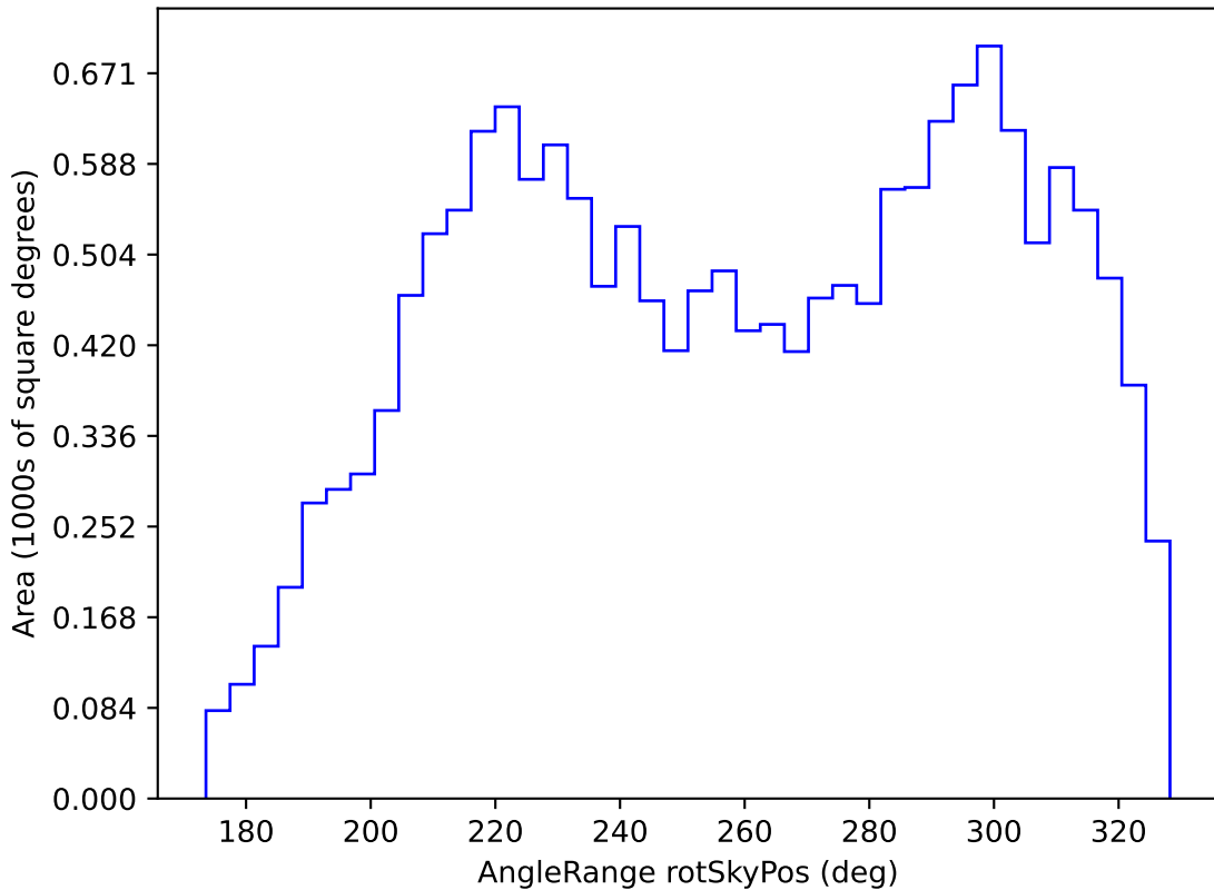
baseline_v3.3_10yrs WFD u band: AngleRange rotSkyPos
