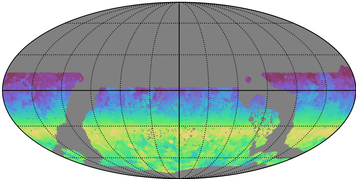
baseline_v3.3_10yrs WFD r band: AngleRange rotSkyPos
