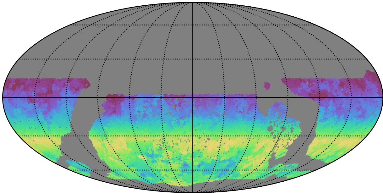
baseline_v3.3_10yrs WFD i band: AngleRange rotSkyPos
