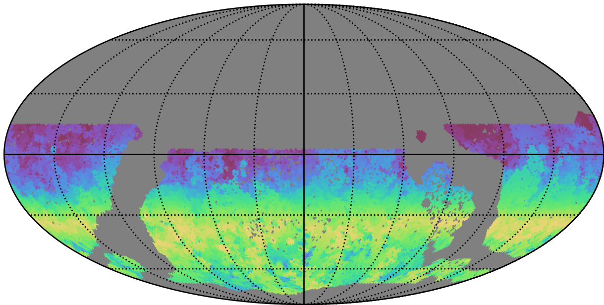
baseline_v3.3_10yrs WFD g band: AngleRange rotSkyPos
