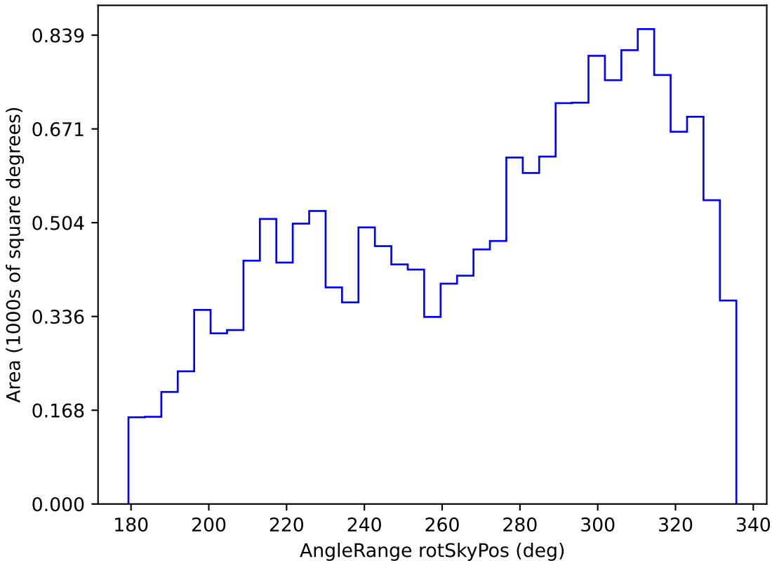
baseline_v3.3_10yrs WFD g band: AngleRange rotSkyPos
