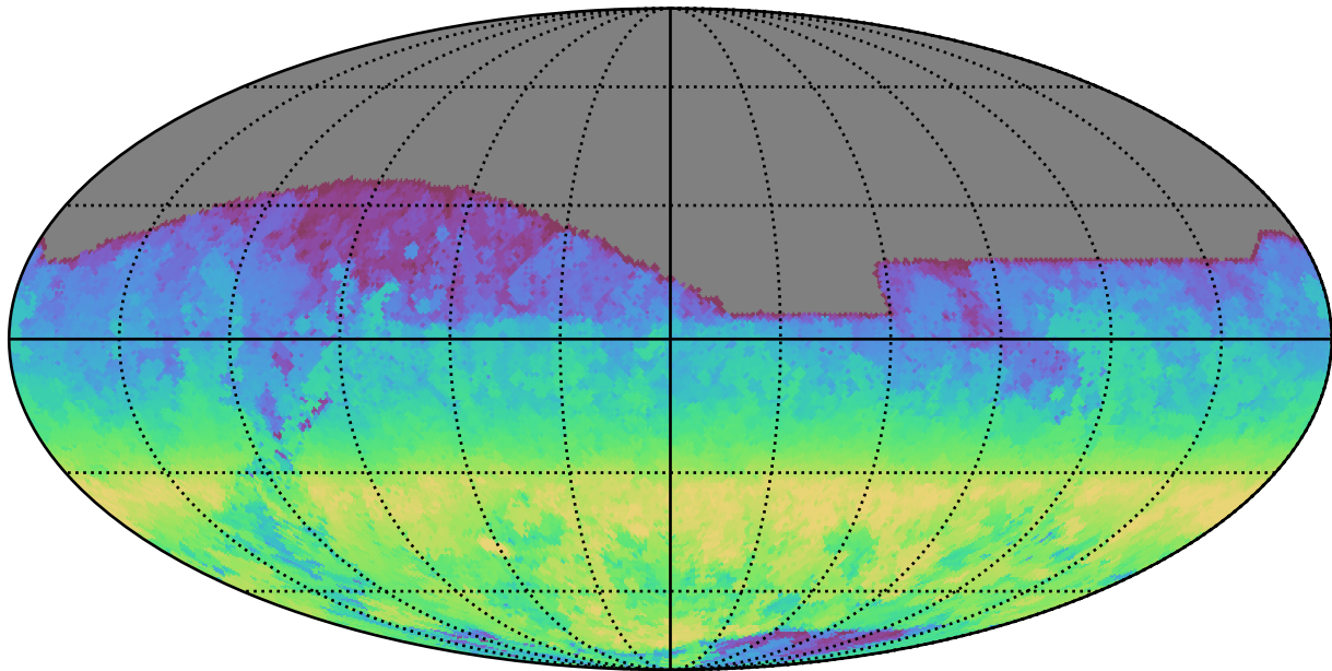
baseline_v3.3_10yrs All sky z band: AngleRange rotSkyPos
