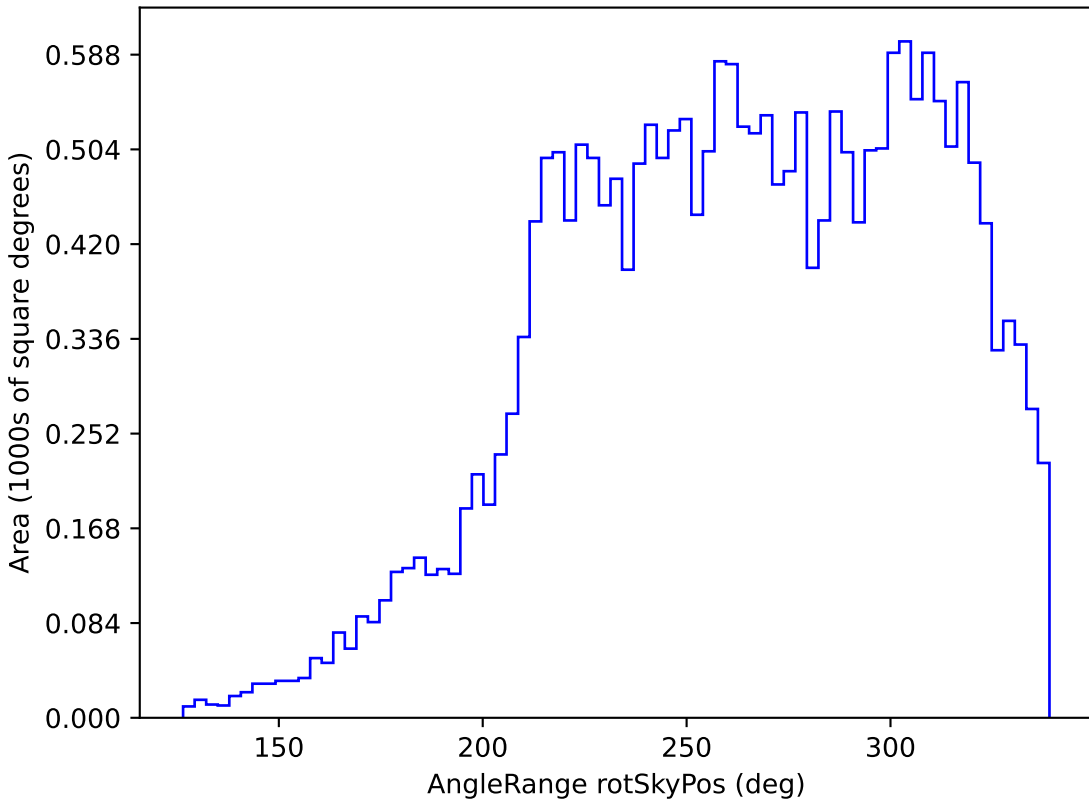
baseline_v3.3_10yrs All sky y band: AngleRange rotSkyPos
