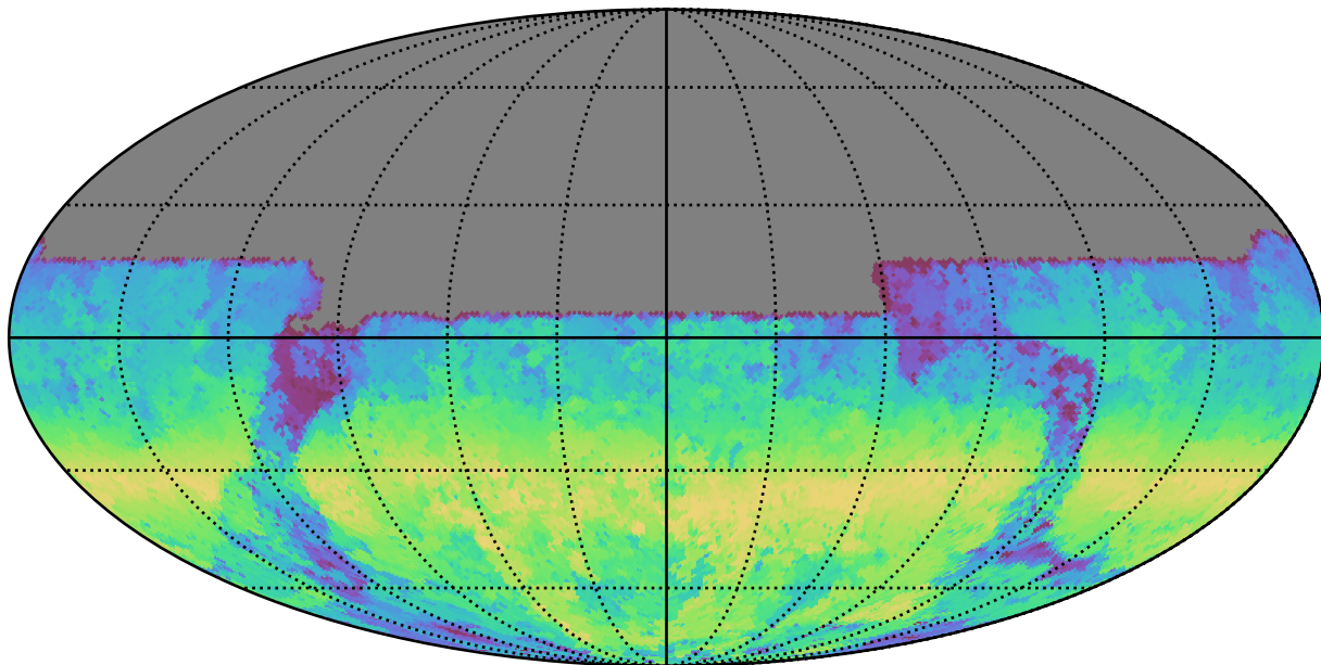
baseline_v3.3_10yrs All sky u band: AngleRange rotSkyPos
